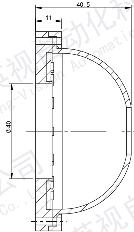
剖面 H-H
